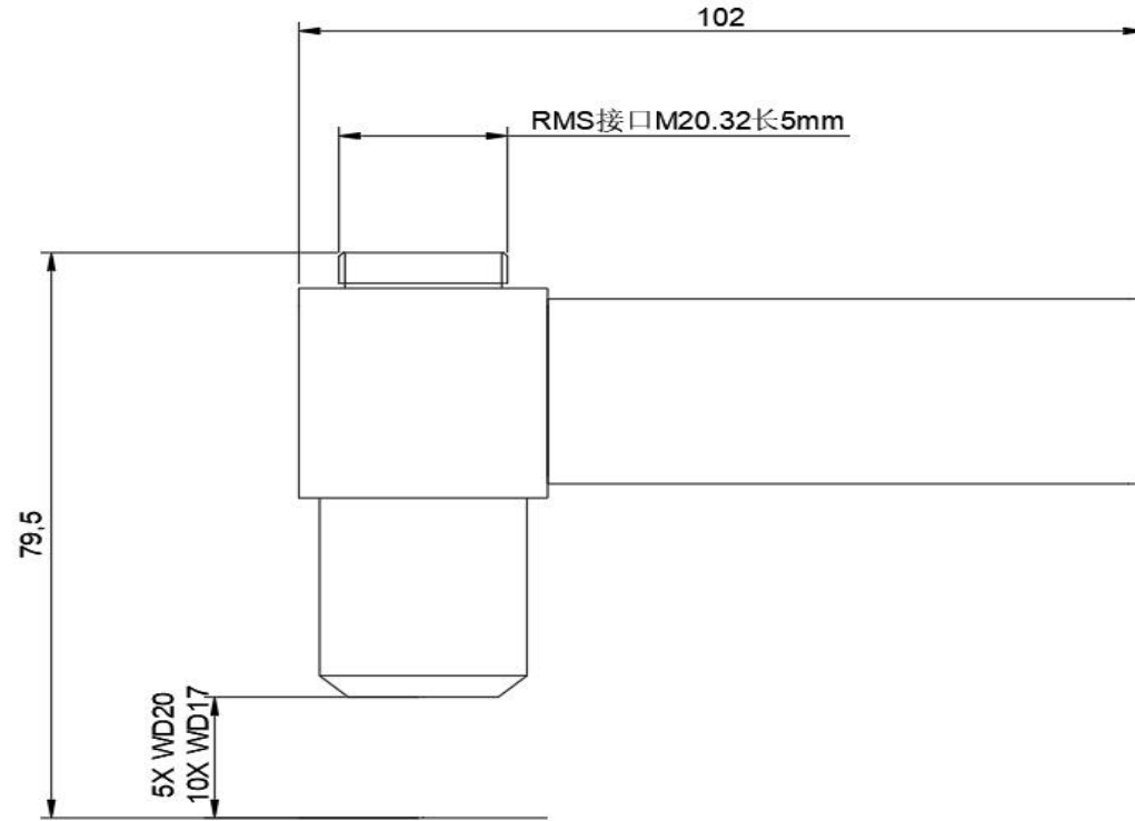
5X,10X Linnik 干涉物镜尺寸图
